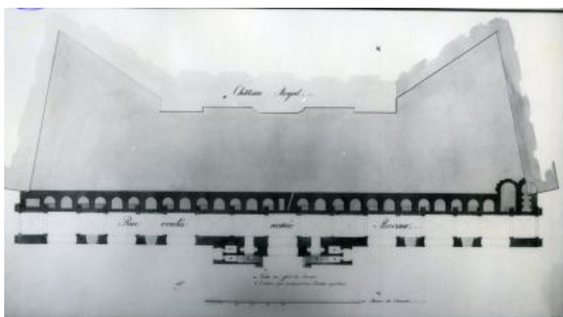
rys.2. Rzut ścian filarów i schodów Arkad z zaznaczonym przebiegiem ul. Bocznej -rysunek projektowy Jakuba Kubickiego z 1817 r.; widoczne pozostawione Stancje Dolne rozebranej Oficyny Tarasowej oraz zarys bryły Zamku; wł. Archiwum Główne Akt Dawnych
