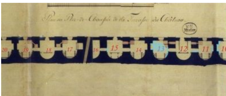
rys.3. Rzut przyziemia Oficyny Tarasowej (tzw. Stancje Dolne) – fragment środkowy z odrestaurowanymi Stancjami 13-14 (sień i izba), rezerwatem architektonicznym (pierwotnie sień-stancja 15), „kątem na drwa wedle kanału” i kanałem odpływowym; wł. Gabinet Rycin BUW
