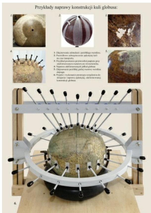
rys.3. Przykłady naprawy konstrukcji kuli globusa
